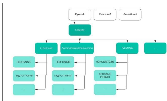
Рисунок 1 Структура портала
