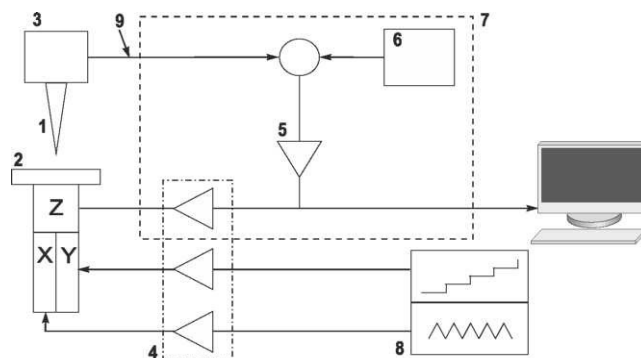
Сурет 1. Сканерлейтін зондты микроскоптың жалпы сызбасы.
