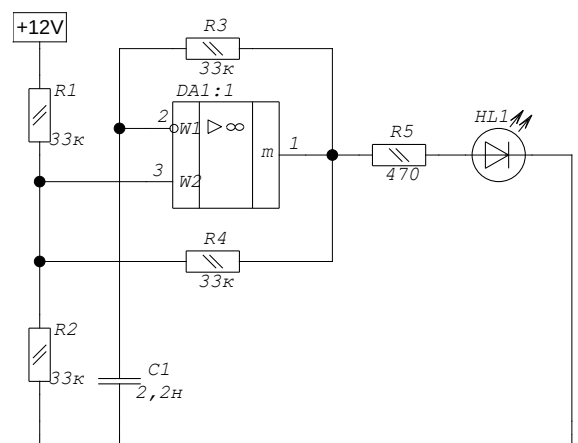
Рисунок 2. Схема электрическая генератора прямоугольных импульсов с излучающим светодиодом
