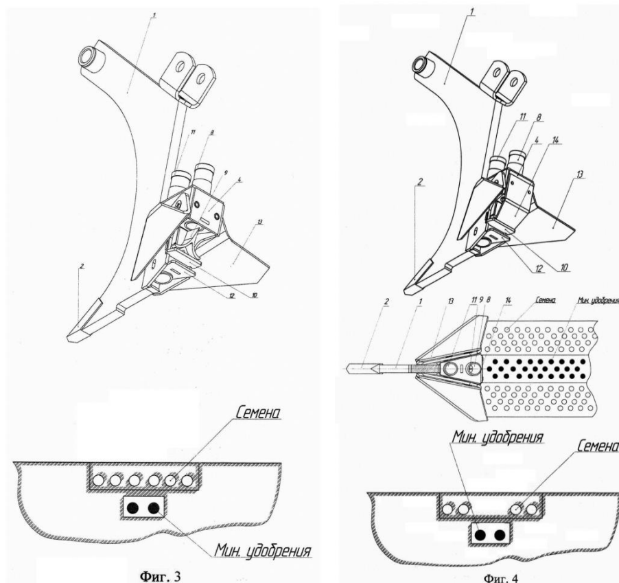
Рисунок 2. Технологическая схема комбинированного сошника для разноуровневого посева семян и внесения удобрений (Патент № 192762): 1 – стойка; 2 – долото; 3 – уступ; 4 – приемник–распределитель; 5, 6, 7, 12 – крепежные пластины; 8 – семянаправитель; 9 – распределитель семян; 10 – отражательная пластина; 11 – тукопровод; 13 – культиваторные лезвия; 14 – съемная пластина
