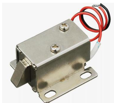
Рисунок 3. Электромеханический замок
