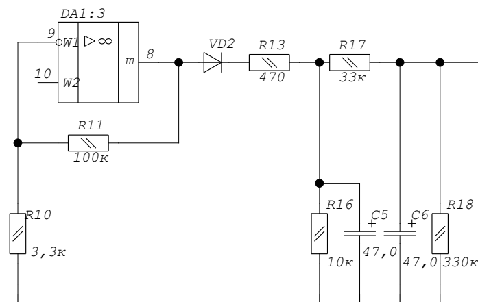
Рисунок 4. Схема электрическая амплитудного детектора и фильтра низкой частоты
