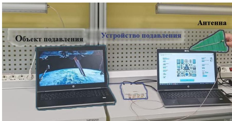
Рисунок 2. Фрагмент эксперимента по радиоэлектронному подавлению
