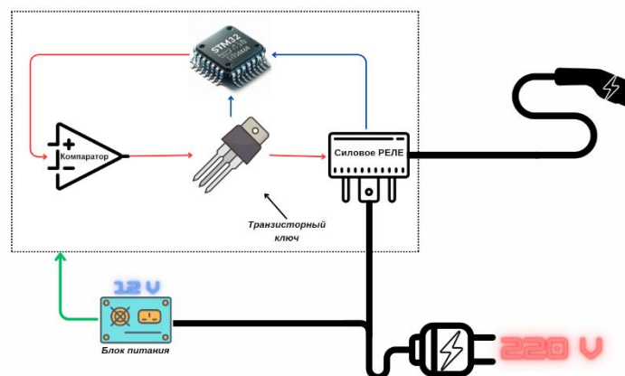
Рисунок 2. Схема модернизации ЗУ
