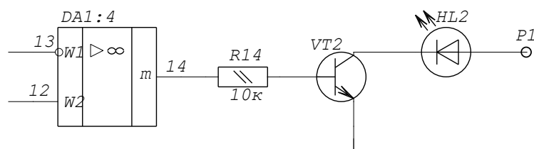
Рисунок 5. Схема электрическая компаратора напряжения
