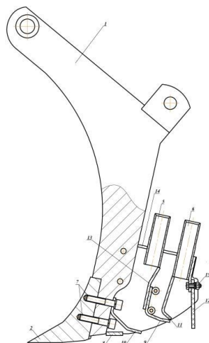
Рисунок 3. Сошник для разноуровневого посева и внесения удобрений (Патент № 204018); 1 – стойка; 2 – плуг; 3 – культиваторные лезвия; 4 – приемник–распределитель; 5 – туконаправитель; 6 – семянаправитель; 7 – болтовое соединение; 8, 9 – пластины уплотнители; 10, 11 скатные пластины; 12 – отражательная пластина; 13 – разделительная пластина; 14 – крепежная пластина; 15 – болтовое соединение
