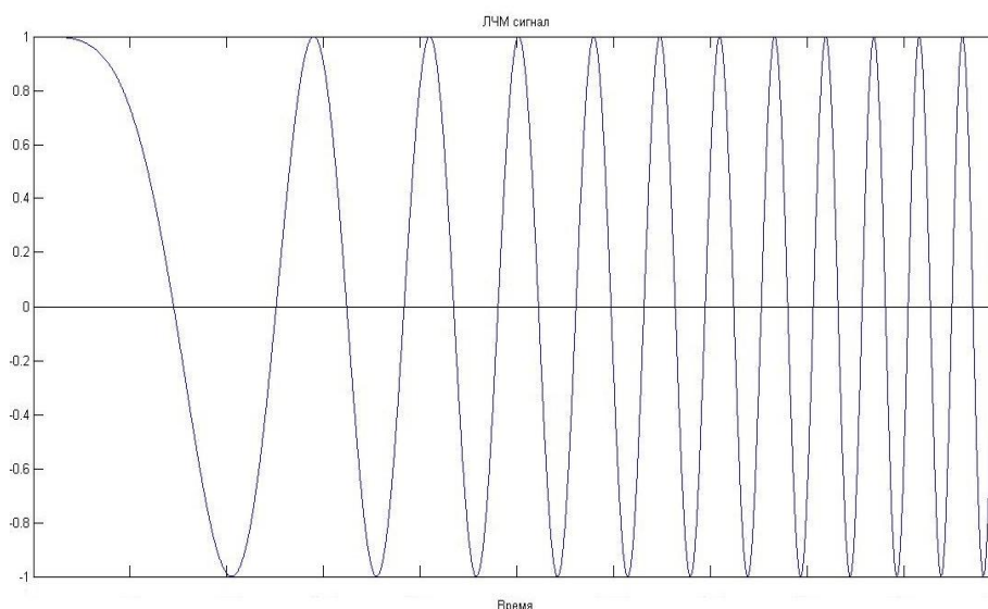
Рисунок 1. Сигнал ЛЧМ (CSS)
