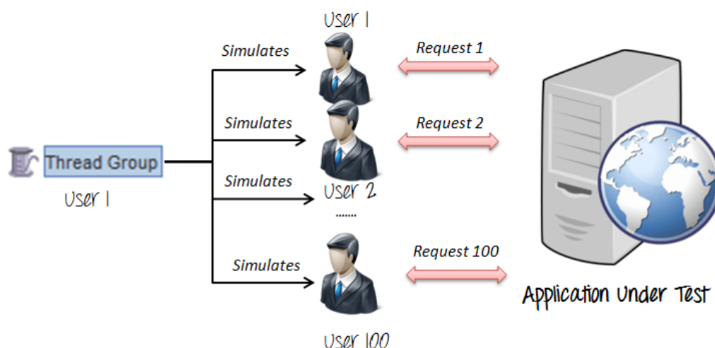
Рисунок 1. Процесс нагрузочного тестирования с использованием JMeter
