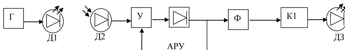
Рисунок 1. Структурная схема устройства определения фотометки с автоматической настройкой контрастности
