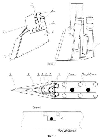
Рисунок 1. Технологическая схема комбинированного сошника для разноуровневого посева семян и внесения удобрений (Патент № 183148): 1 – долото; 2 – крепежная пластина; 3 – стойка; 4 – семянаправители; 5 – туконаправитель; 6 – расширители; 7 – уплотнительная пластина
