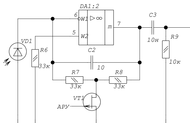
Рисунок 3. Схема электрическая преобразователя тока фотодиода в напряжение с усилителем с АРУ
