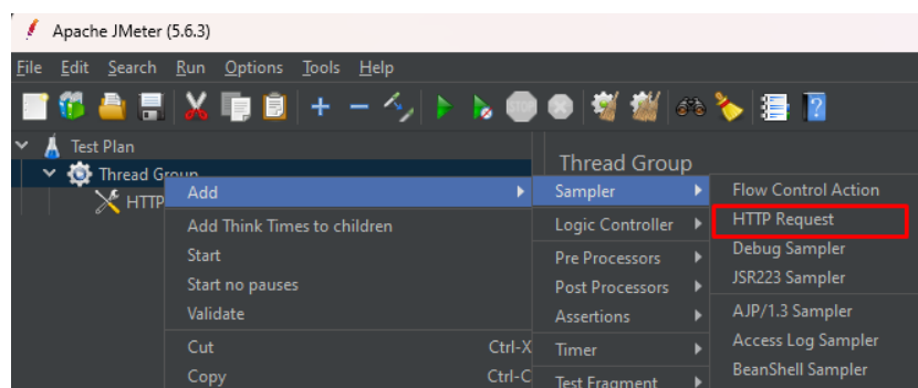
Рисунок 6. Создание компонента HTTP Request
