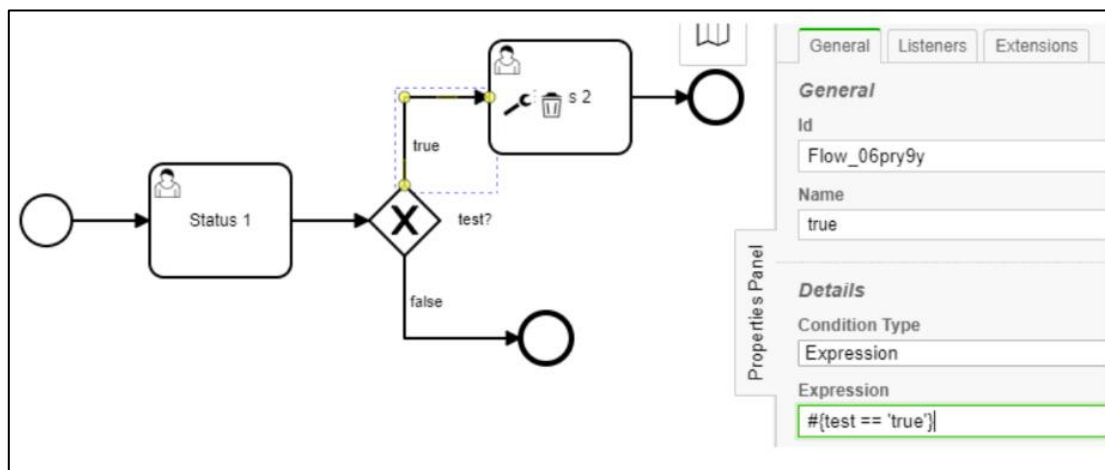
Рисунок 1. Пример доработки блока путем внедрения кода
