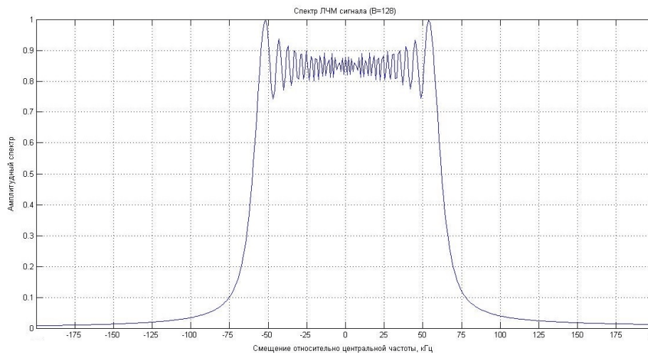
Рисунок 2. ЛЧМ спектр
